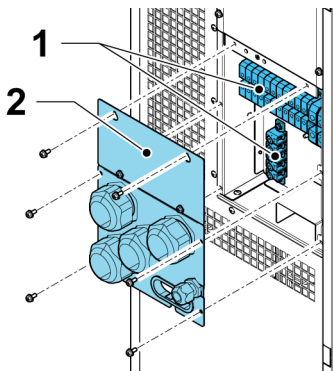
Рисунок 12: Сальниковая панель и расположение выходов
