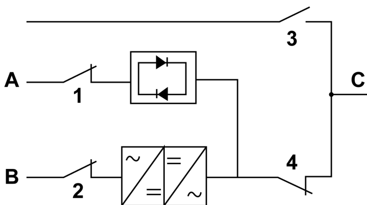
Рисунок 37: Нормальные положения переключателей
