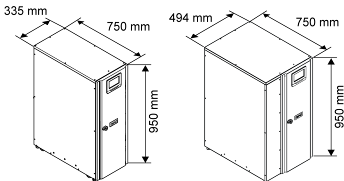
Рисунок 9: Габариты ИБП Eaton 91PS/93PS 8–10 кВт с приставкой и без нее
