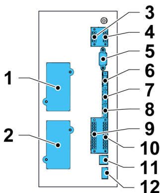
Рисунок 23: Интерфейсы связи на раме ИБП 91PS/93PS 8–10 кВт
