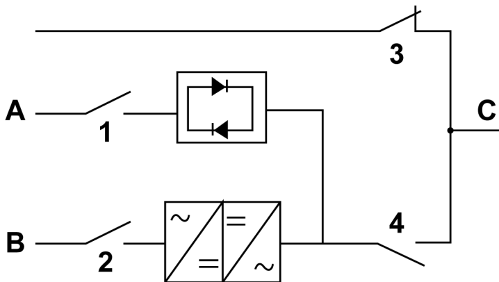
Рисунок 36: Режим сервисного байпаса
