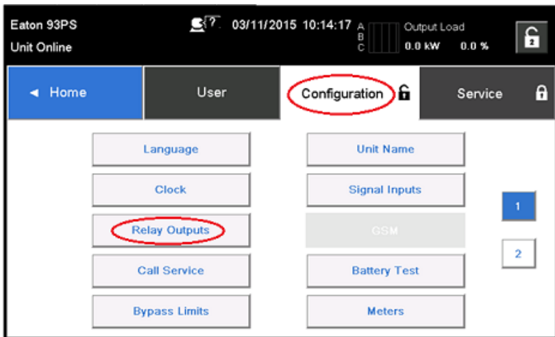
Рисунок 29: Выбор пункта Выходы реле в экране Конфигурация
