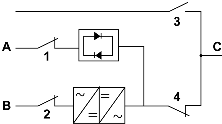
Рисунок 34: Нормальные положения переключателей
