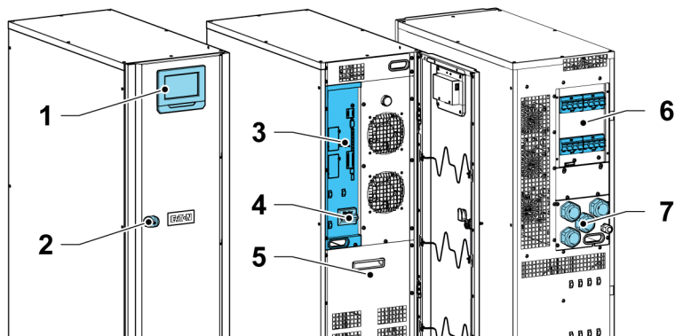
Рисунок 2: Компоненты ИБП Eaton 91PS/93PS 8–10 кВт внутри стандартной рамы
