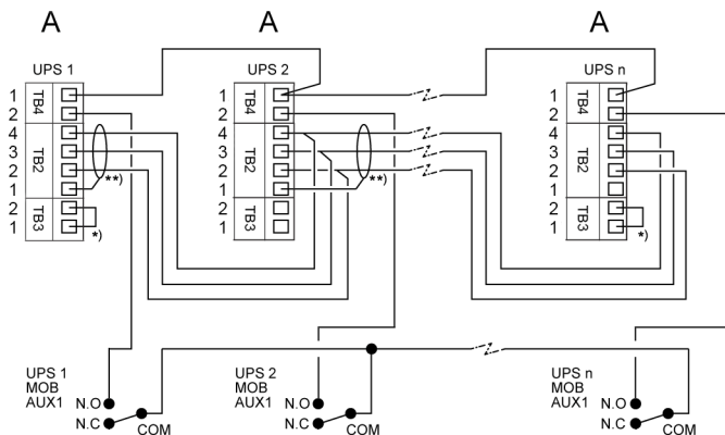
Рисунок 21: Проводка для сети CAN и параллельного монтажа для системы ИБП с параллельным подключением и выходными выключателями модулей
