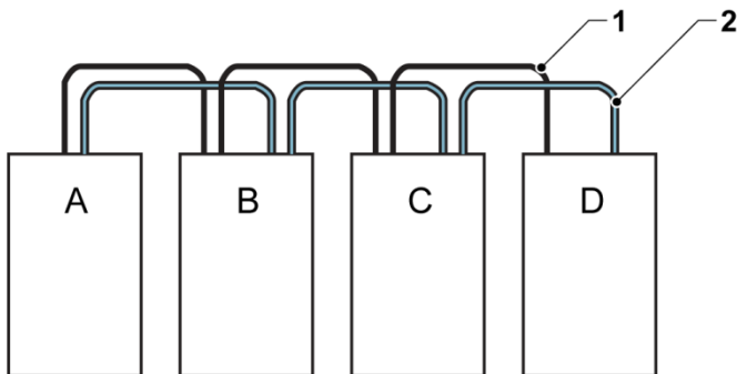
Рисунок 20: Упрощенная схема проводки для сети CAN и проводки «Pull chain» для системы ИБП с параллельным подключением
