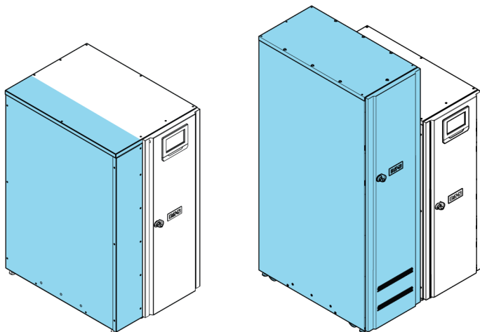
Рисунок 16: ИБП 91PS/93PS 8–10 кВт с опциональным аккумуляторным шкафом/аккумуляторной приставкой (слева)
