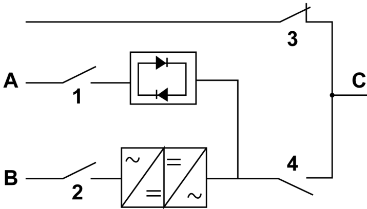
Рисунок 35: Режим сервисного байпаса
