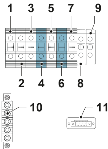
Рисунок 11: Клеммы для подключения силовых кабелей ИБП для однофазных блоков
