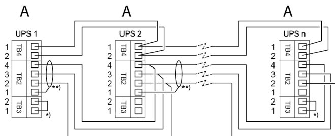
Рисунок 22: Проводка для сети CAN и параллельного монтажа для системы ИБП с параллельным подключением без выходных выключателей модулей
