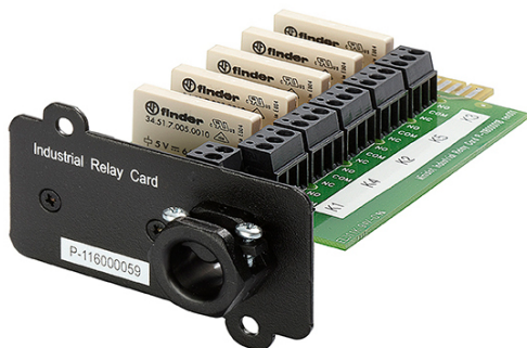
Рисунок 27: Карта промышленного реле - MS
