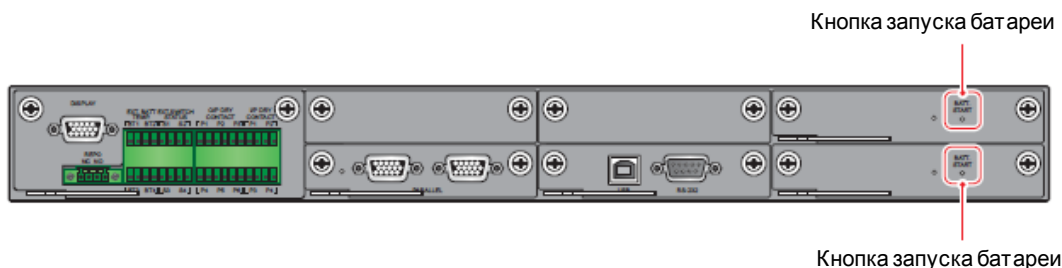
Рисунок 4-17: Расположение кнопок запуска батарей
