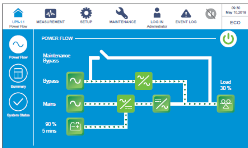
Рисунок 6-26: Экран ECO-режима
