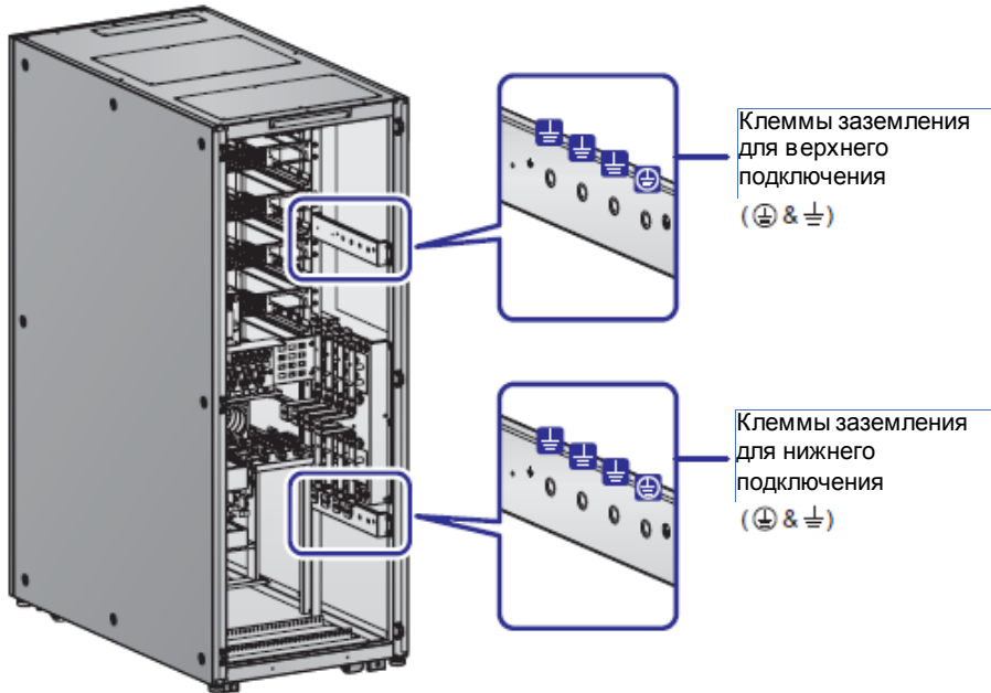
Рисунок 5-13: Клеммы заземления
