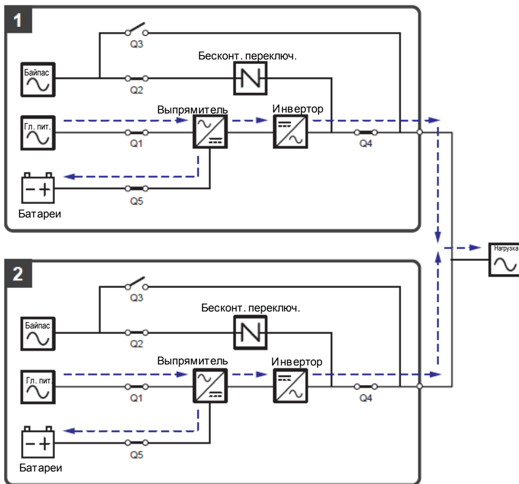
Рисунок 3-28: Схема режима преобразования частоты, подключение параллельных ИБП к двум линиям
