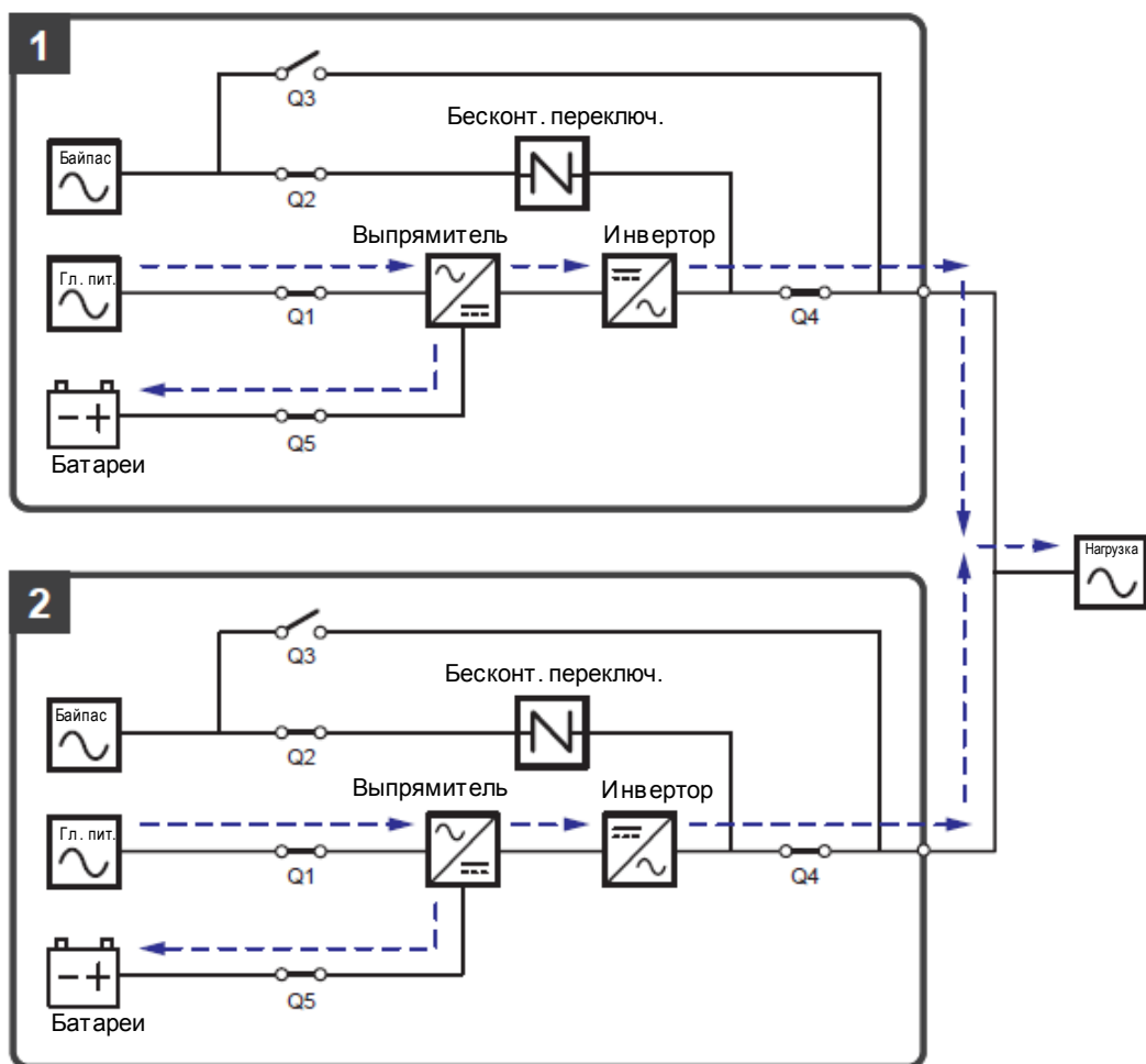
Рисунок 3-23: Схема режима двойного преобразования, подключение параллельных ИБП к двум линиям
