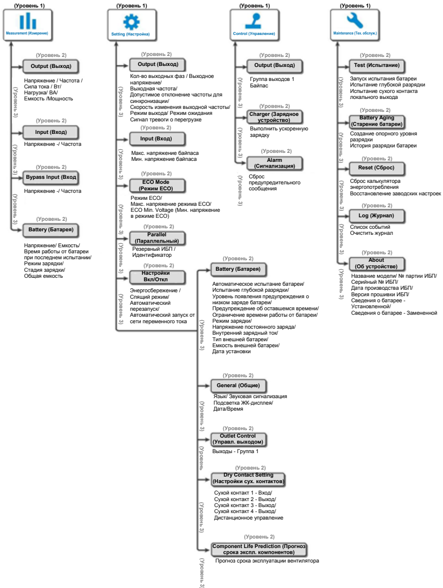
Рисунок 9-1: Дерево меню
